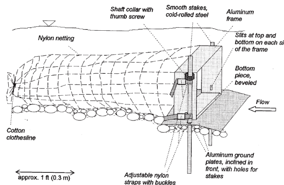
Figure 19: Bedload trap (Bunte et al. 2007).
